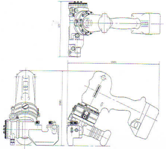
外観寸法図(mm)
